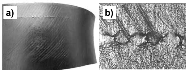
Rys. 5. Rozwarstwienia na bocznej powierzchni próbki, widok: a) makroskopowy, próbka nr 4, b) rozwarstwienia na granicy zgrzanych metali, pow. 25× Fig. 5. Delamination on the side surface of the specimen, view: a) the macroscopic, specimen no. 4, b) delamination at the border line between explosion welded metals, magn 25×
