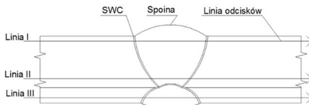
Rys. 6. Przekrój złącza spawanego z naniesionymi liniami pomiaru twardości
