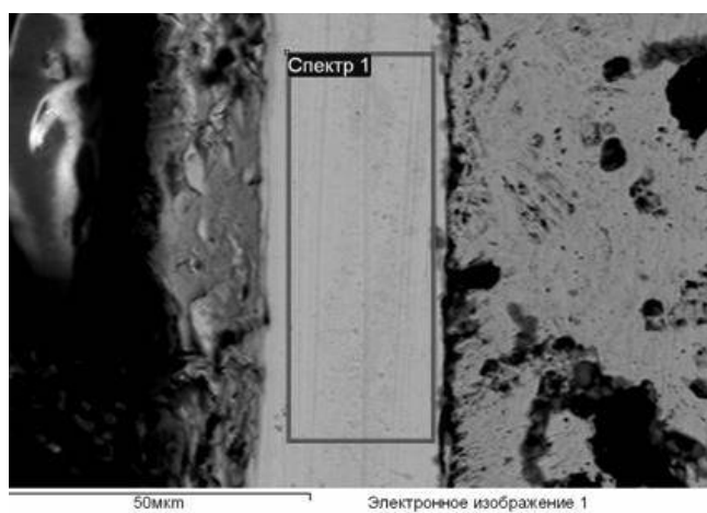
Рис. 2 – Структура склад нанесеного покриття
