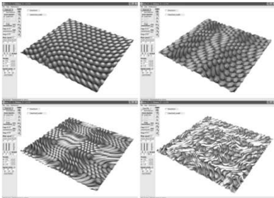
Рис. 9 – Варіанти розрахованої простої та складної асиметричної інтерпольованої перфорованої структури для підвищення енергетичного обміну в турбулентизованих середовищах
