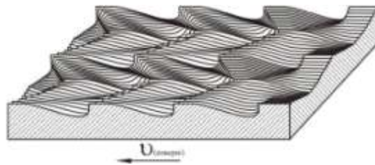
Рис. 5 – Варіант складної порції поверхні з урахуванням перетікання при заданій турбулізації потоку для збільшення енергообміну з середовищем
