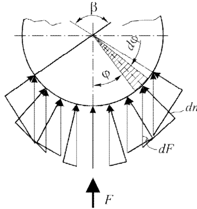
Рис. 2 □ Распределение нормальных сил по дуге обхвата колодочной детали
