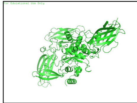
Gambar 2. Struktur Protein Glutathione S Transferase P (Sumber: Dokumen Pribadi melalui Pymol)
