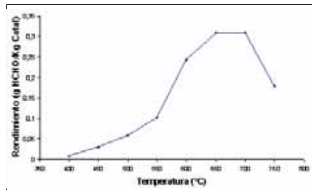
Figura 4. Rendimientos de HCHO catal. Fe 0,5%/SiO 2
