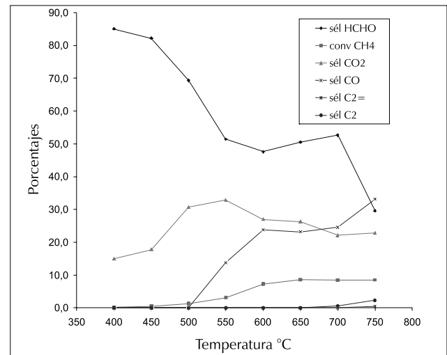
Figura 3. Selectividades de productos y conversión de CH 4 para el catalizador de Fe 0.5%/SiO 2
