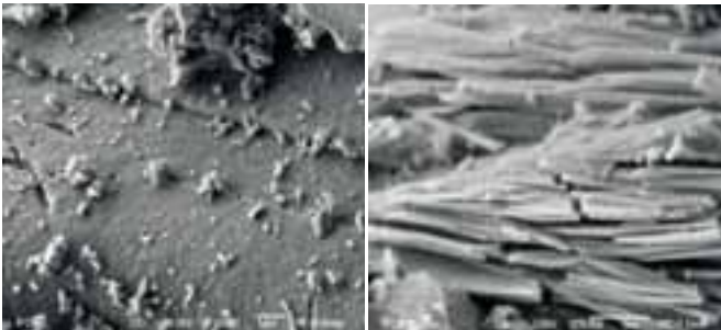
Foto 7. Catalizador 7 (0.5%Fe/SiO 2 ) Foto 8. Catalizador 5 (0.4%Fe/SiO 2 )
