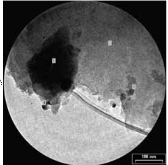
Foto 9. TEM catalizador 6 (Fe 0,5%)
