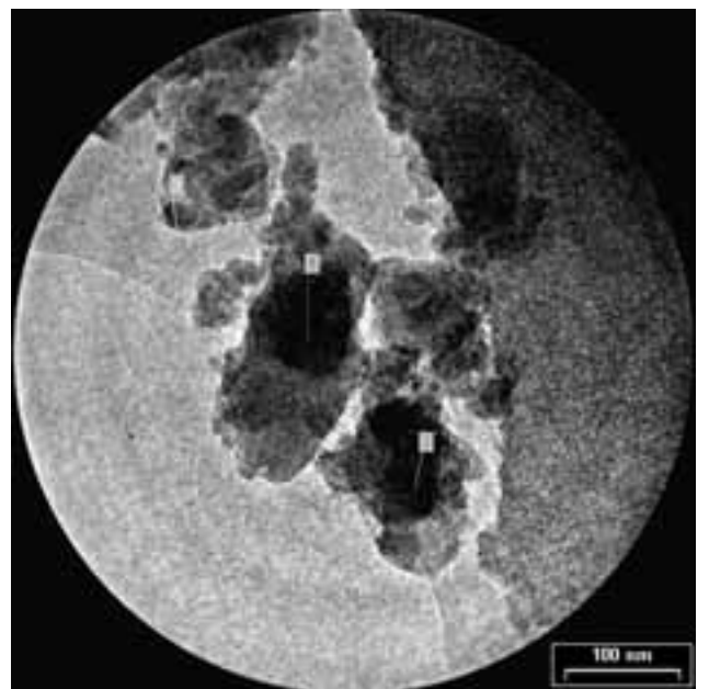
Foto 10. TEM catalizador 7 (Fe 0,5%)
