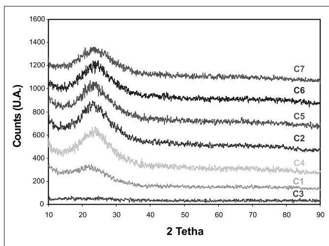
Figura 2. Difractograma de los catalizadores de Fe/SiO 2
